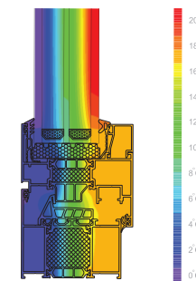
XCLUSIVE 86i 2 Multilock Διάγραμμα Ισοθερμικής Ροής
