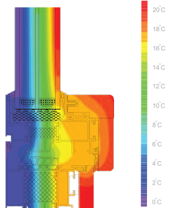
XCLUSIVE 87i 2 Αλουμίνιο + Ξύλο Διάγραμμα Ισοθεμικής Ροής
